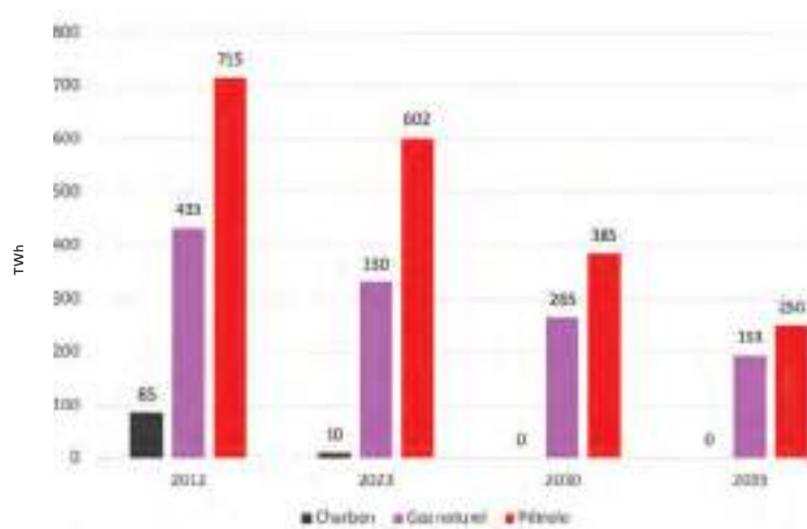
Figure 4. Consommation primaire d'énergies fossiles pour les usages énergétiques historique (2012, 2023) et projetée (2030, 2035) (en TWh, périmètre hexagone (avec Corse), hors soutes internationales, hors consommations de charbon pour la filière fonte) – source : SDES (avril 2025), DGE (dernière version à date du scénario de la Stratégie française énergie-climat)
